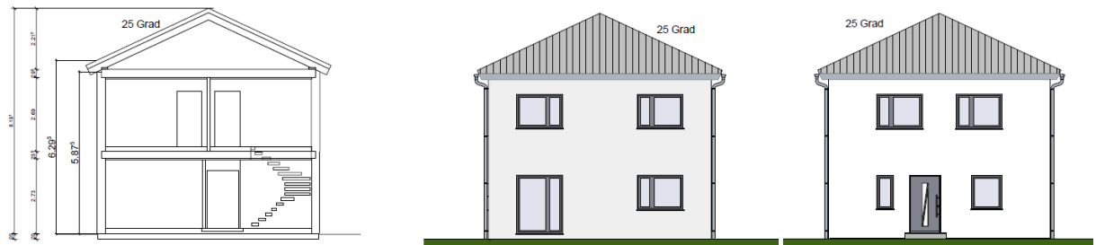
Schnitt, Ansicht Ost und Ansicht West (CEO Rietz Planungsgesellschaft GmbH, 01/2025)
